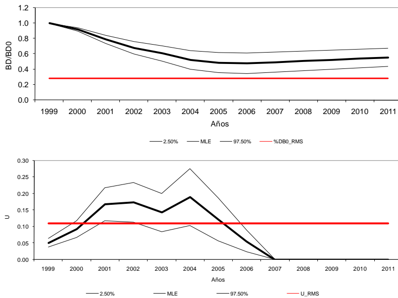
Figura 9. Estimados máximos verosímiles (MLE) e intervalos de confianza al 95% para la razón de agotamiento (BD/BD0) y la tasa de explotación. Las líneas rojas indican los niveles en que se estima se alcanza el rendimiento máximo sostenido. Tomado de Payá (2013).
