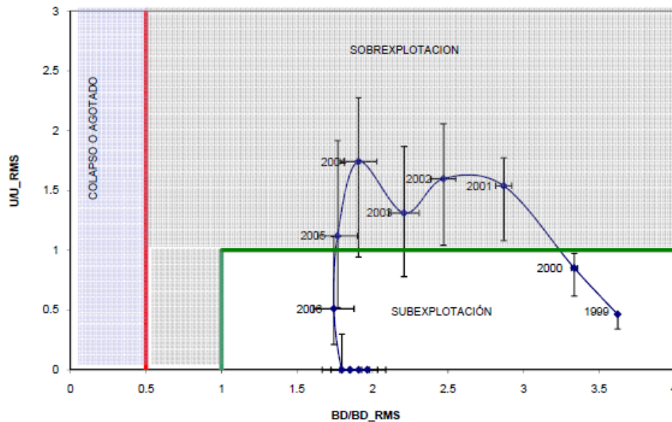
Figura 1. Diagrama de fase que presenta el estatus del stock de ORH. Tomado de Payá (IFOP, 2013).
