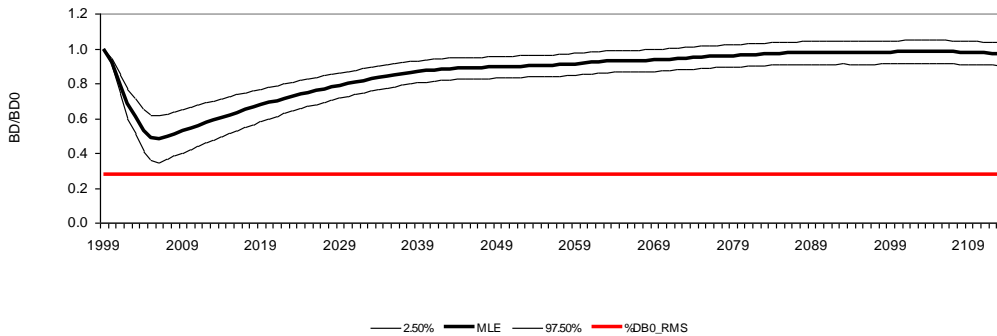
Figura 12. Proporción de la biomasa desovante virginal en las proyecciones de recuperación con veda.
