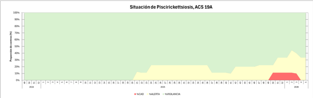
Figura N° 2: Proporción de centros según categoría, PSEVC–Piscirickettsiosis, ACS 19A. (Fuente: Sernapesca).
