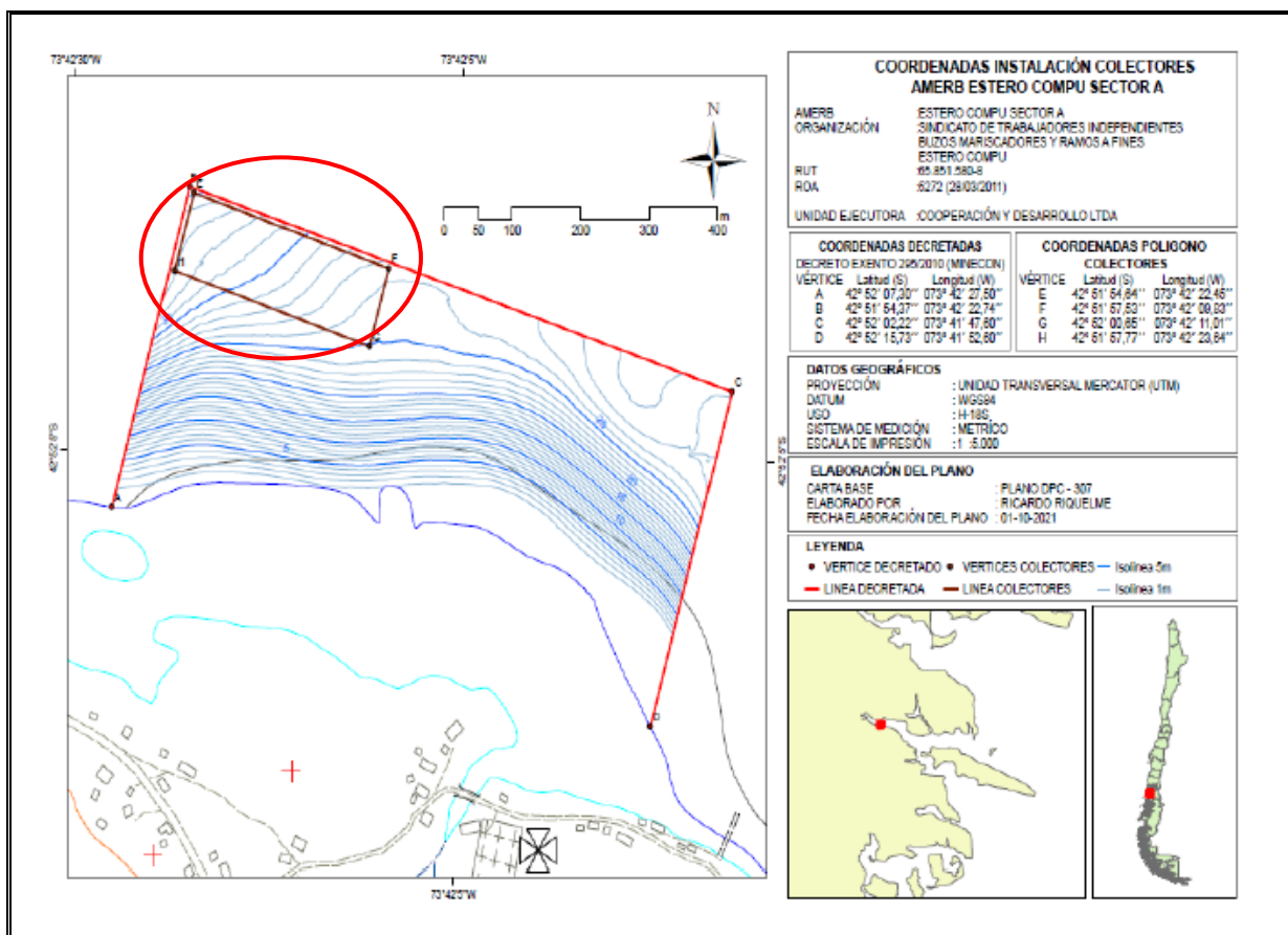
Figura 1. Ubicación del polígono solicitado y visado por Capitanía de Puerto, para la instalación de 15 líneas dobles con colectores de chorito al interior del AMERB "ESTERO COMPU SECTOR A" , Región de Los Lagos.
