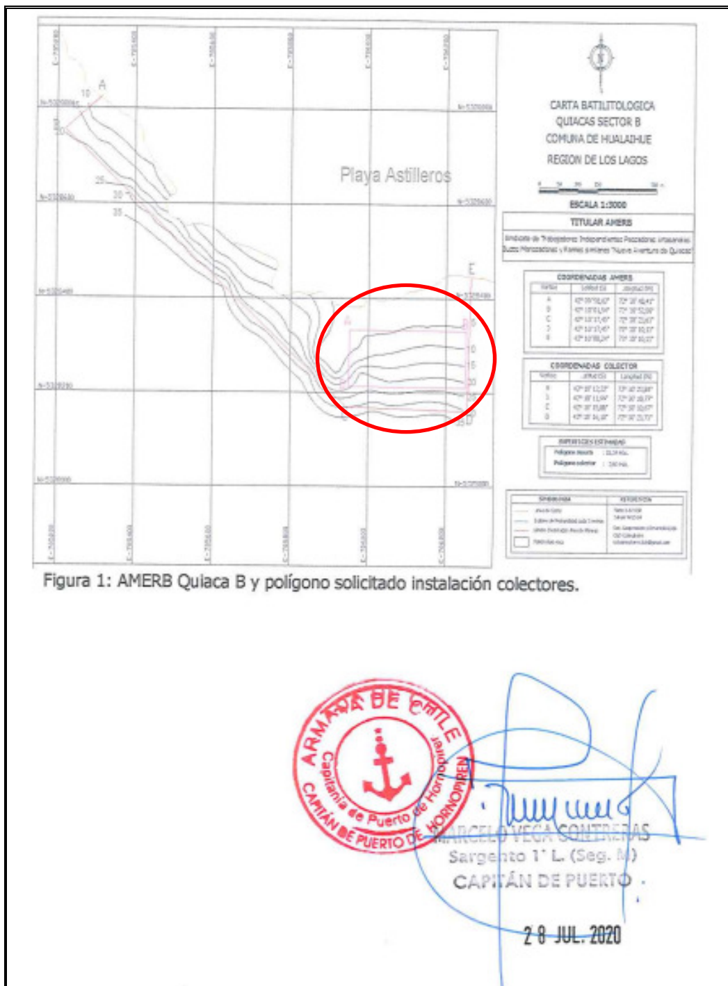
Figura 1. Ubicación de polígono solicitado y visado por Capitanía de Puerto, para la instalación de 14 líneas dobles con colectores de chorito al interior del AMERB “Quiacas sector B”, Región de Los Lagos.
