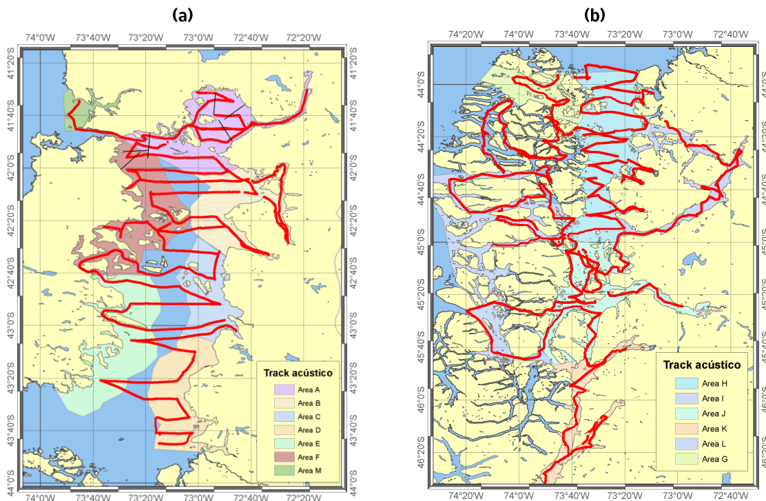
Figura 10. Track acústico por áreas de evaluación (Dic 2010 - Ene 2011): (a) X Región de Los Lagos y, (b) XI Región de Aysén. (Fuente: Cubillos et al. 2011).
