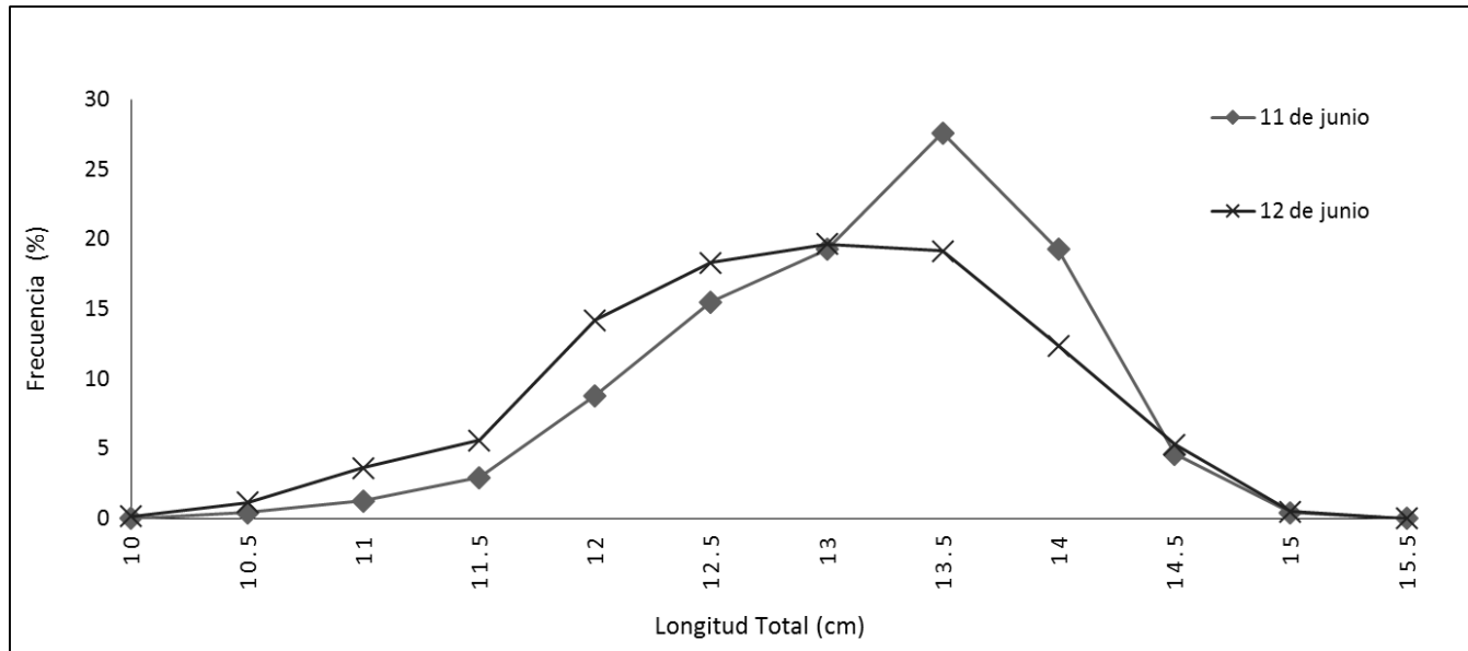
Figura 1. Estructura de tallas de anchoveta en la Zona de Antofagasta. Sábado 11 y domingo 12 de junio, 2016.
