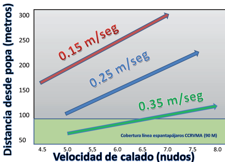
Figura.2. Efecto combinado de la velocidad de calado y la tasa de hundimiento de la línea madre sobre la distancia tras popa a la cual los anzuelos alcanzan los 10 metros de profundidad. Se indica la cobertura aérea de una línea espantapájaros (LEP) según los estándares de la CCRVMA (90 metros).
