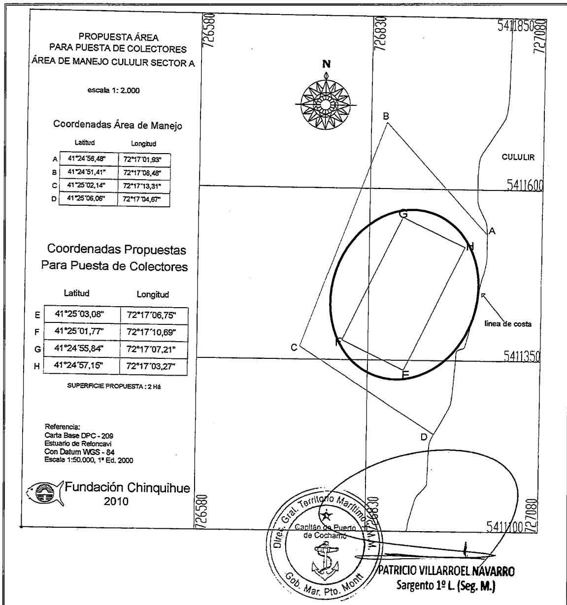
Figura 1. Ubicación del polígono solicitado y visado por Capitanía de Puerto, para la instalación de 6 líneas dobles con colectores de chorito al interior del AMERB "Cululir sector A", Región de Los Lagos.
