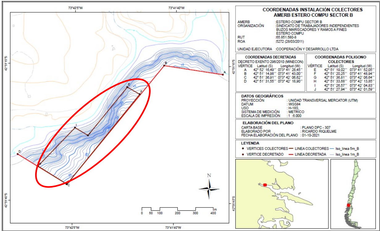
Figura 1. Ubicación del polígono solicitado y visado por Capitanía de Puerto, para la instalación de 23 líneas dobles con colectores de chorito al interior del AMERB "ESTERO COMPU SECTOR B", Región de Los Lagos.
