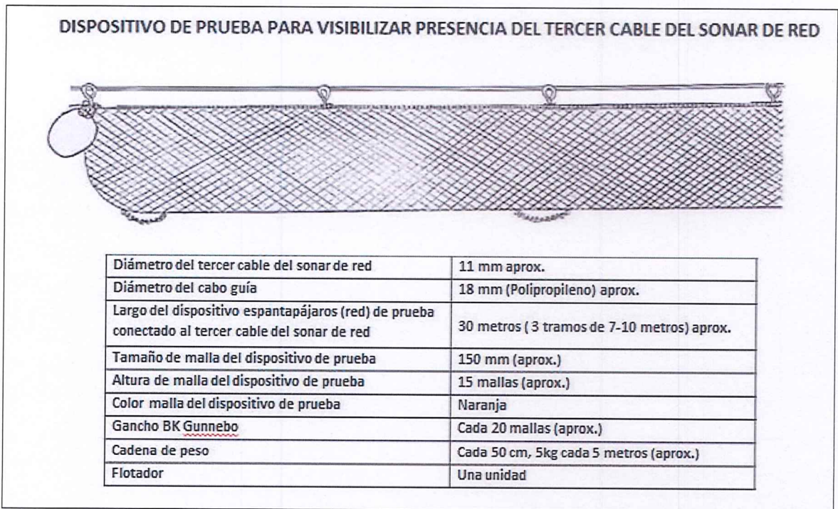
Figura 1: Esquema de dispositivo de prueba para visibilizar la presencia del tercer cable
