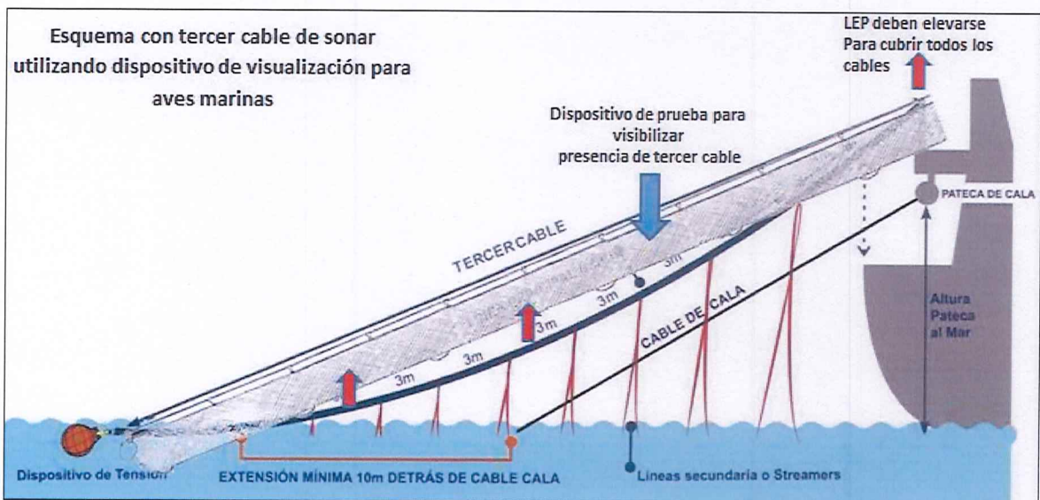
Figura 2: Esquema del tercer cable utilizando dispositivo de prueba para visualización
